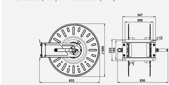
Dimensions (mm) / Dimensioni (mm)
