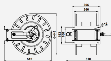
Dimensions (mm) / Dimensioni (mm)
