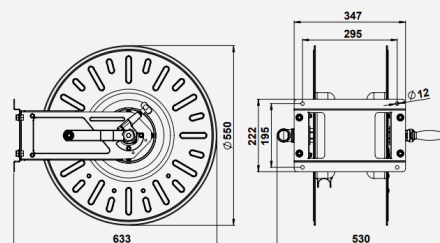
Dimensions (mm) / Dimensioni (mm)
